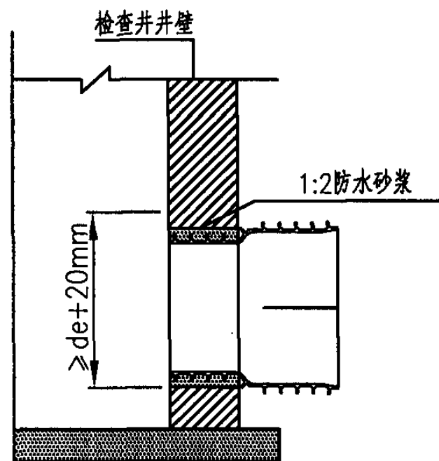
管道与检查井的连接(四)
