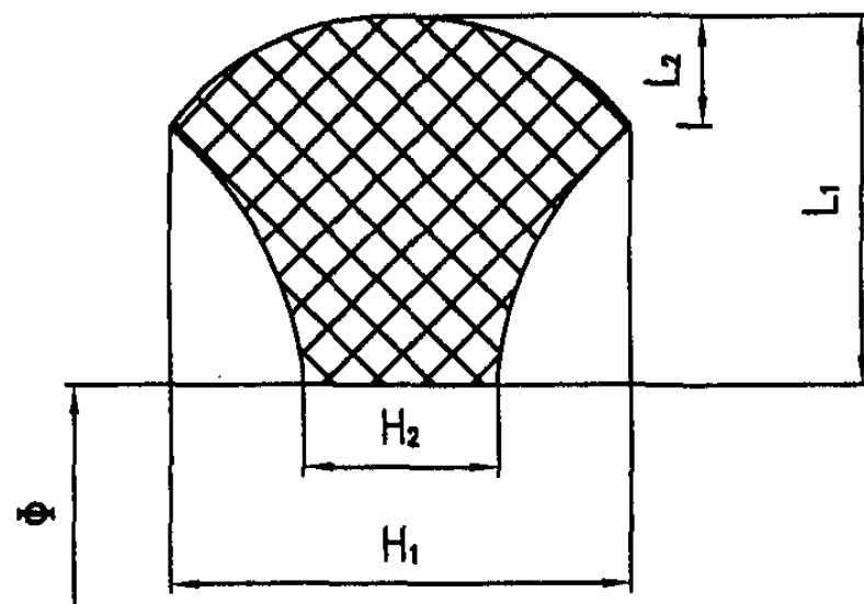
De400~De800橡胶圈截面
