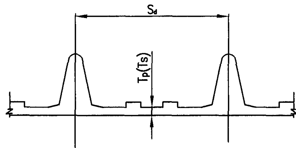
管肋大样图
