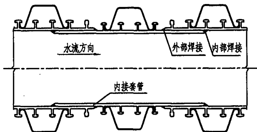
PE钢塑复合缠绕管接口示意图
