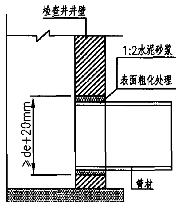
管道与检查井的连接(一)
