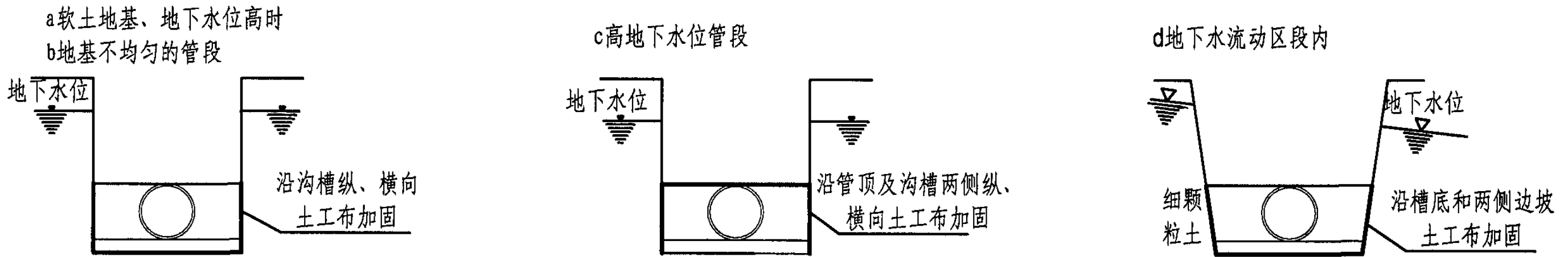
沟槽横断面图
