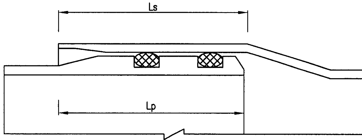
管道接口图
