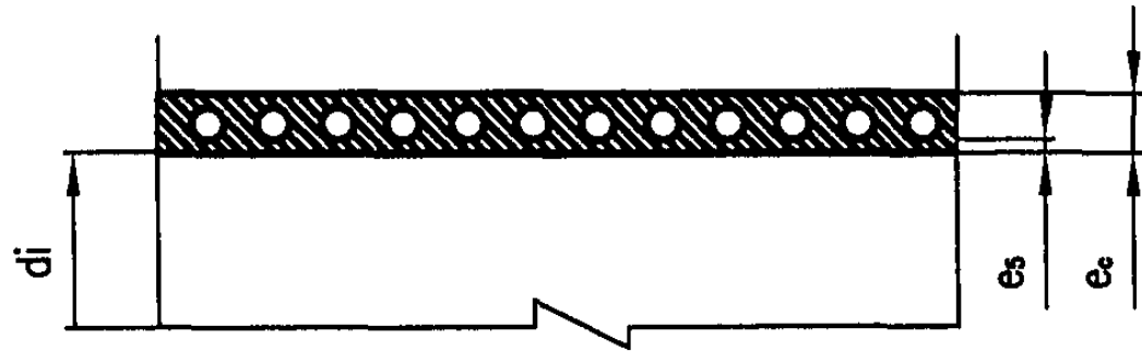
A型结构壁管的典型示例2
