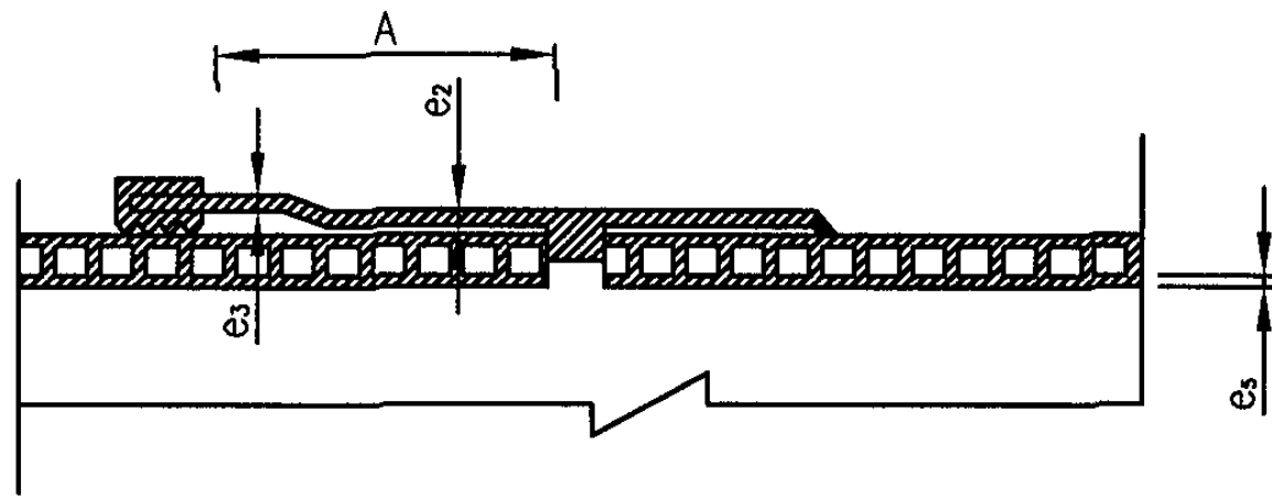
典型弹性密封件接口
