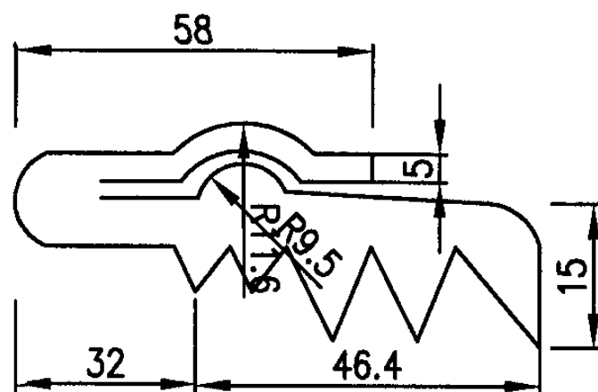
弹性密封件尺寸图
