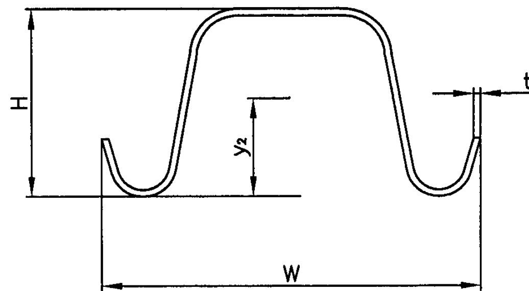
V4型钢肋截面示意图
