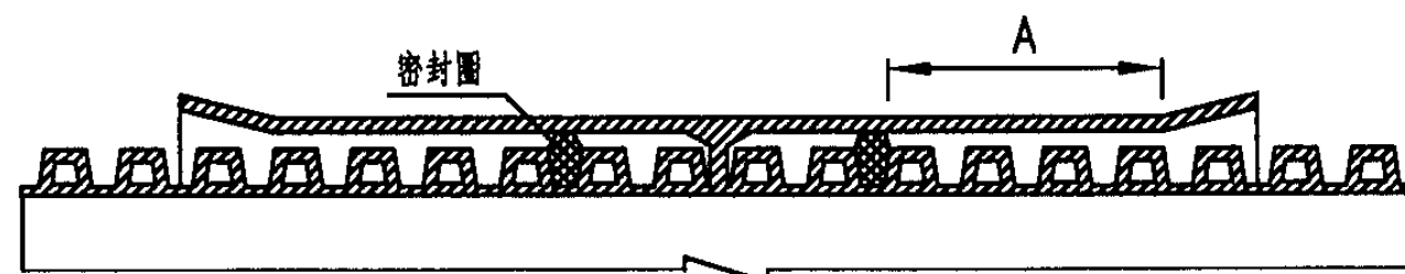
b) 不带扩口管材结构示意图
