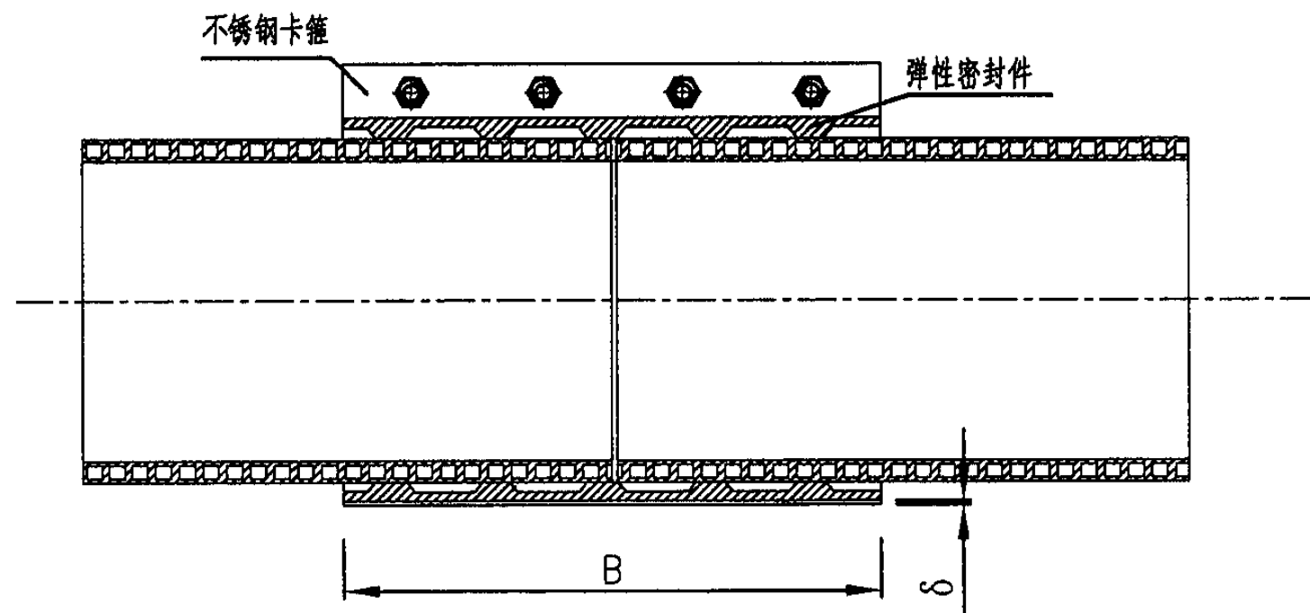
卡箍式弹性密封件接口示意图
