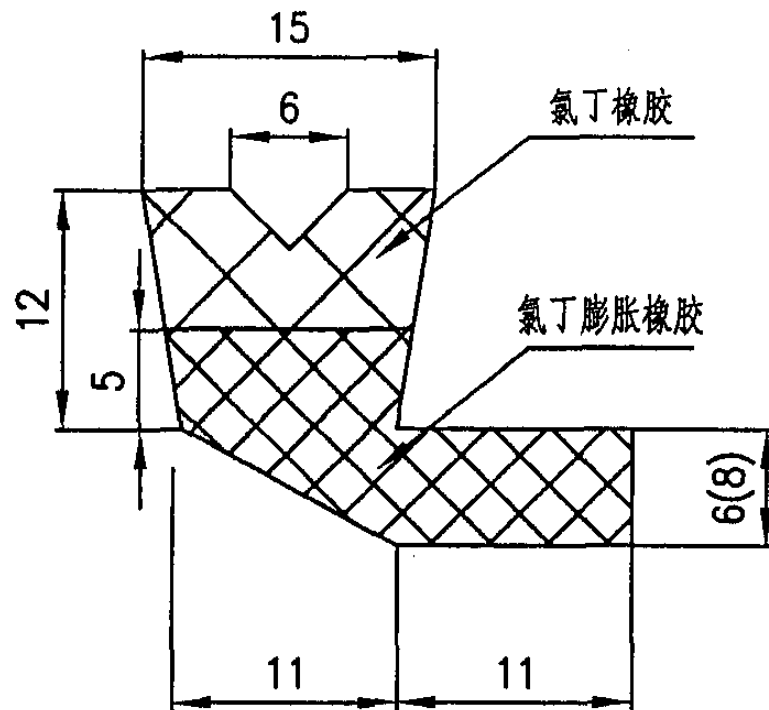
Φ700~800
