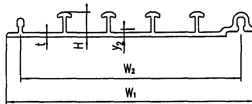
PE板材截面示意图
