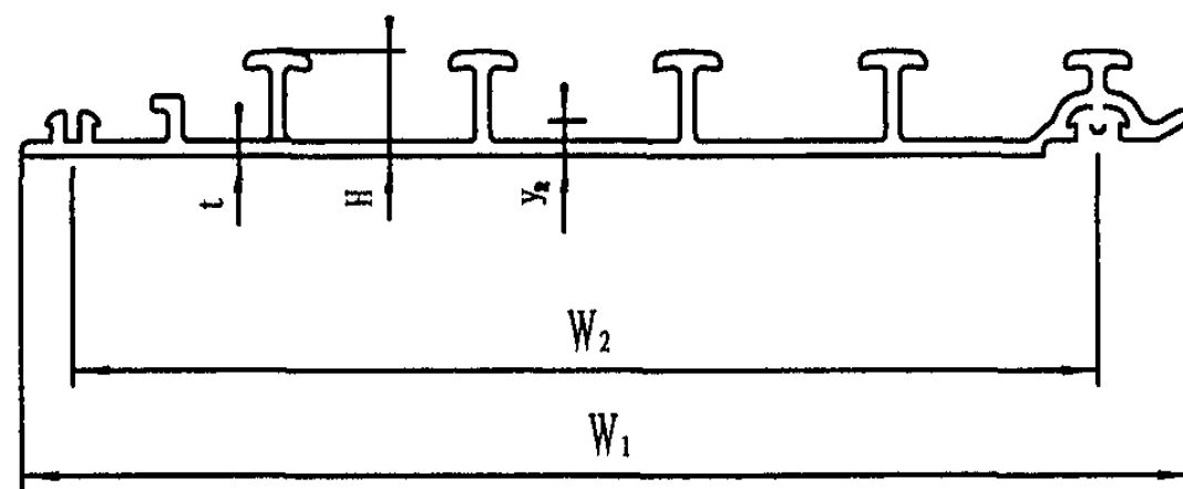
PVC-U板材截面示意图
