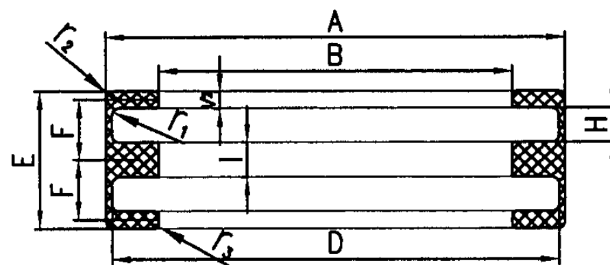
连体密封圈截面
