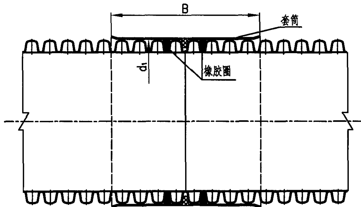
套筒尺寸
