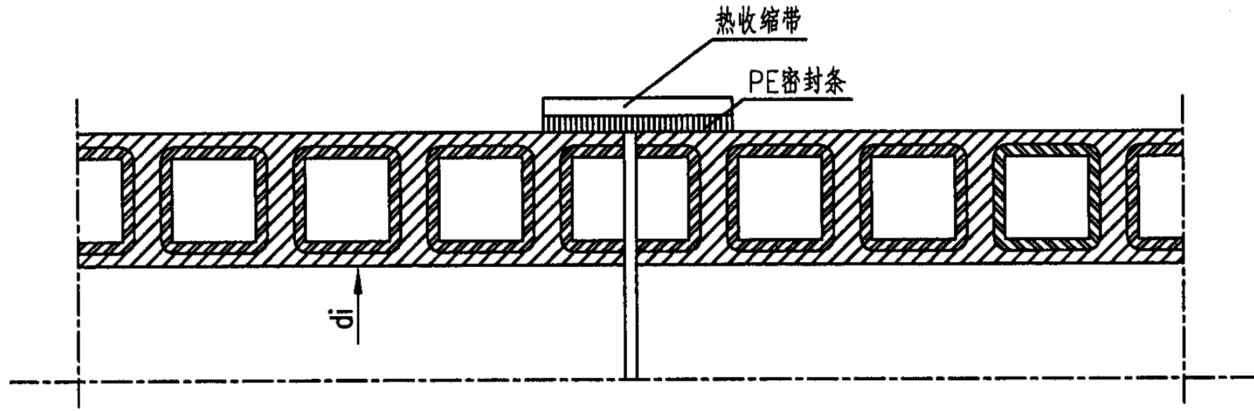
热收缩带接口示意图
