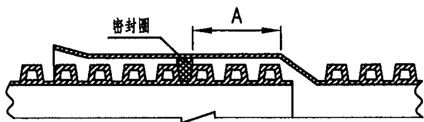
c) 承接式连接示意图
