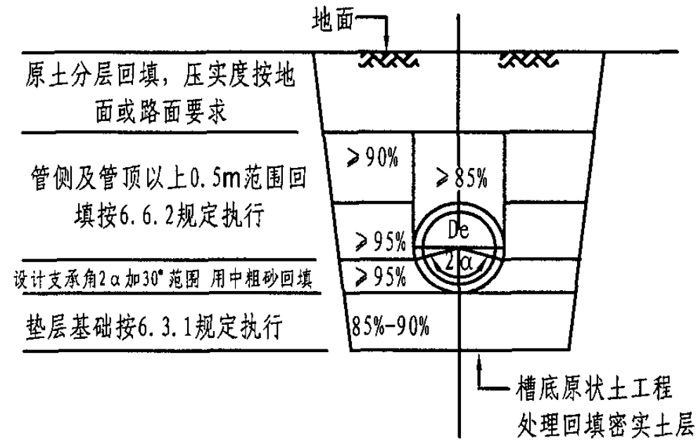
图 1 沟槽回填土压实要求
