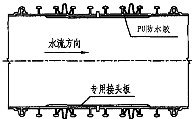
PVC-U钢塑复合缠绕管接口示意图
