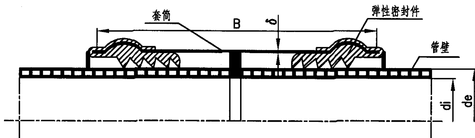
双向承插弹性密封件接口示意图
