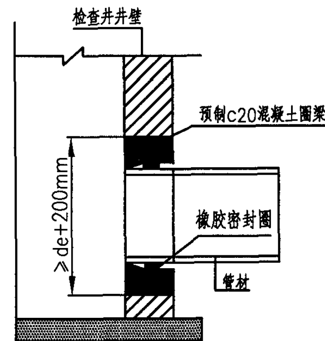
管道与检查井的连接(五)
