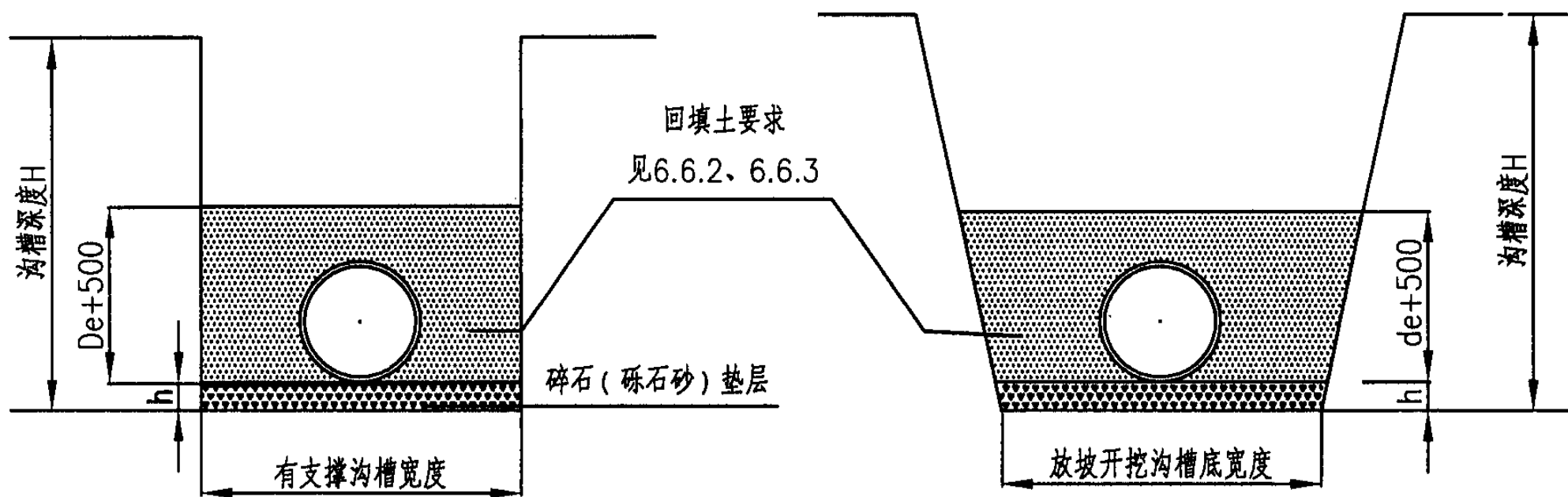
管道基础图
