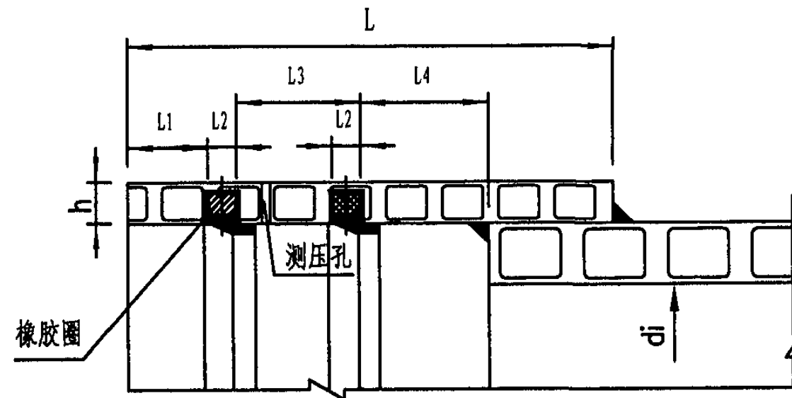
b 污水管道承口(有测压孔)
