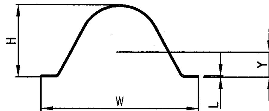
U3型截面示意图
