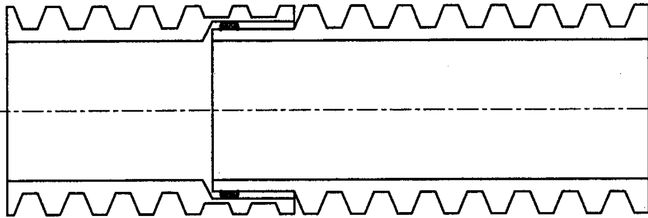
管道接口图
