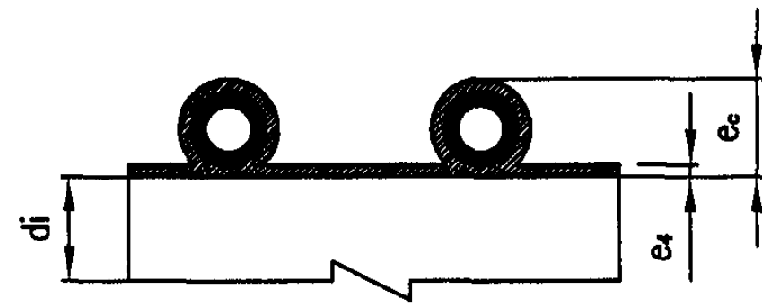
B型结构壁管的典型示例1
