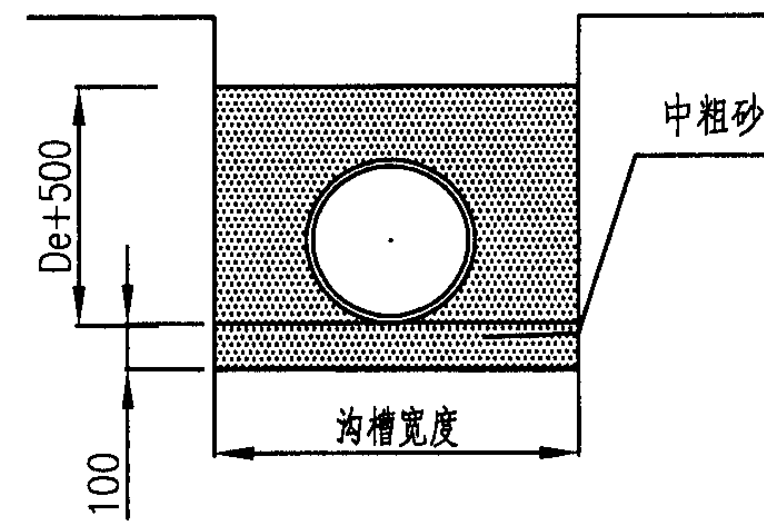
雨水口连接管基础图
