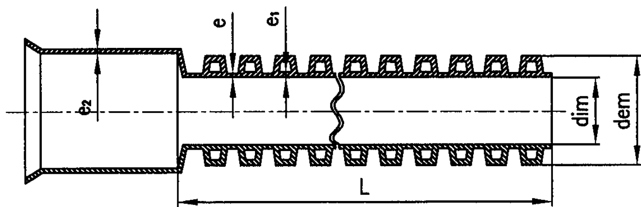
a) 带扩口管材结构示意图
