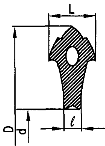
密封圈截面
