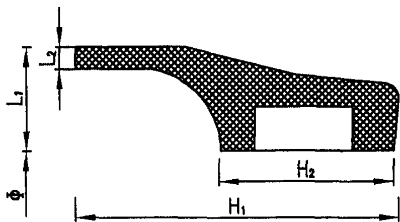
橡胶圈截面
