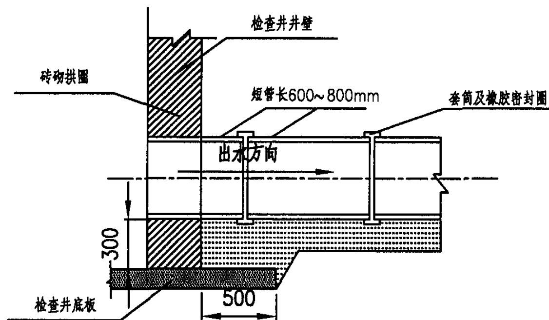
落底检查井
