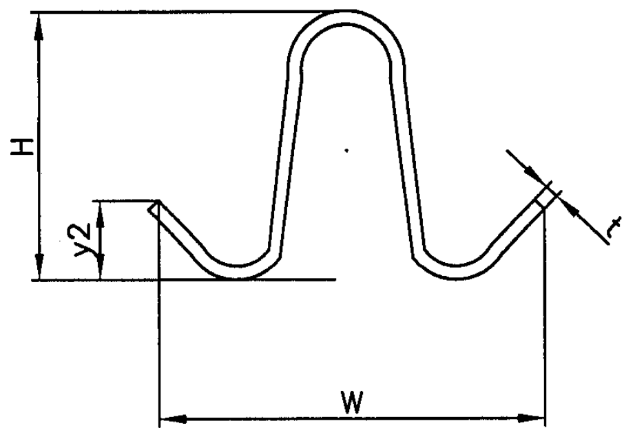
V3型钢肋截面示意图
