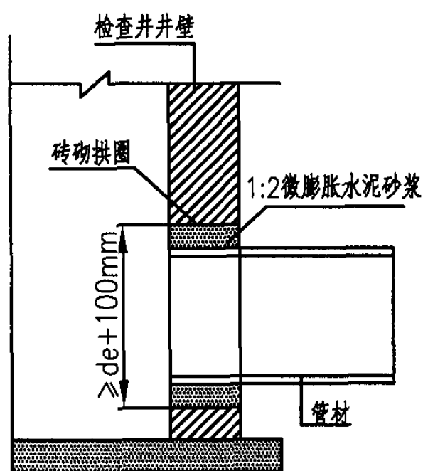
管道与检查井的连接(三)
