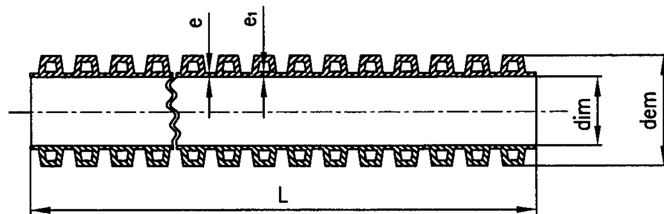
b) 不带扩口管材结构示意图
