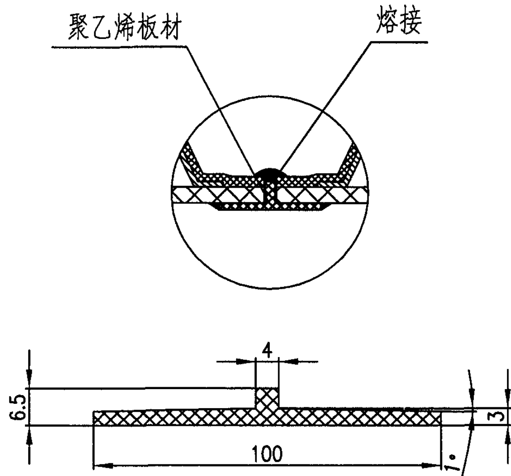
聚乙烯板材尺寸
