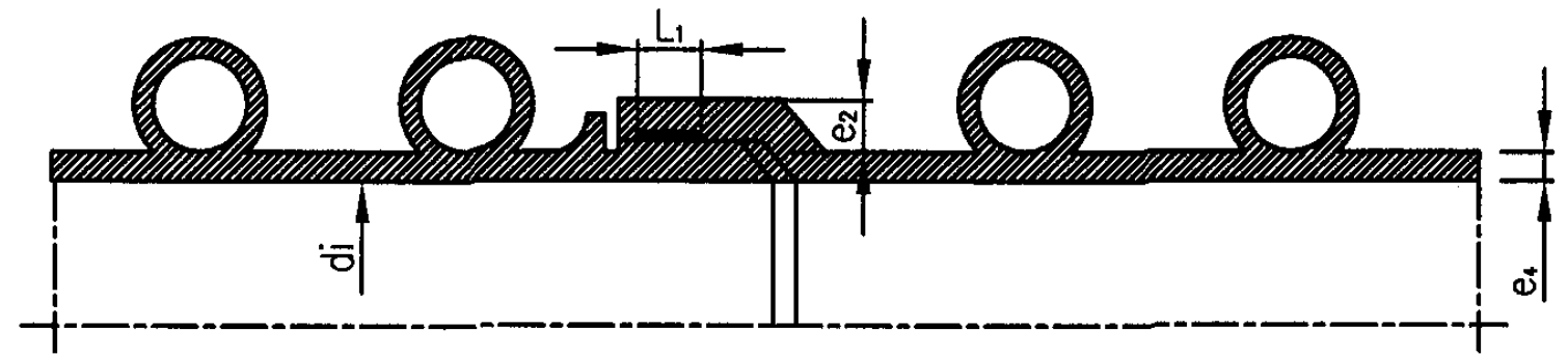
典型承插口电熔连接接口
