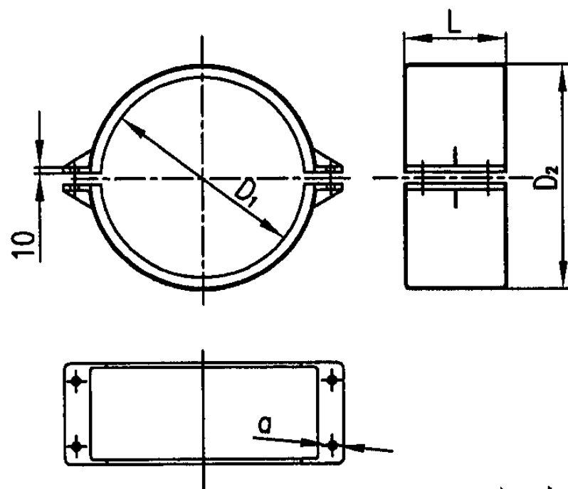
哈夫外箍件图
