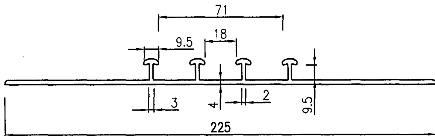
PE内接套管截面尺寸
