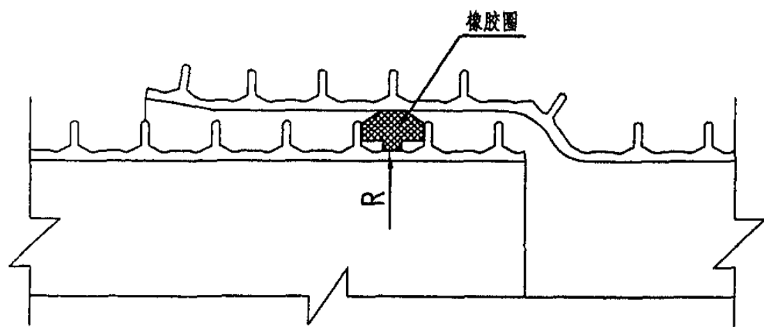
管道接口图
