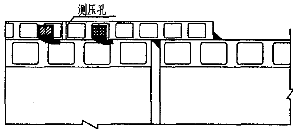
污水承插式接口
