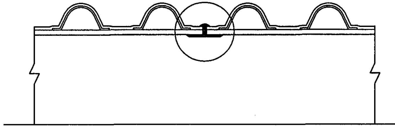
聚乙烯内衬板材焊接接口示意图
