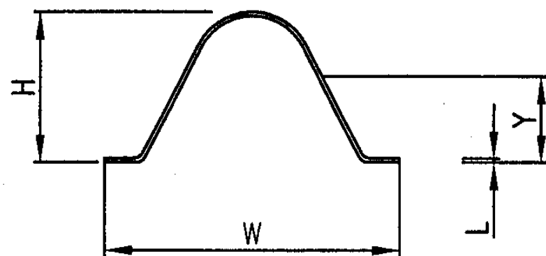
U2型截面示意图
