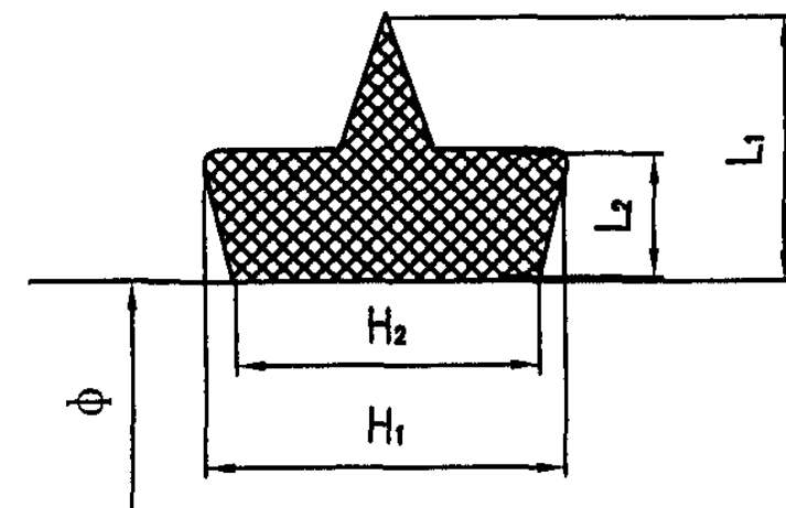
Di200~Di300橡胶圈截面
