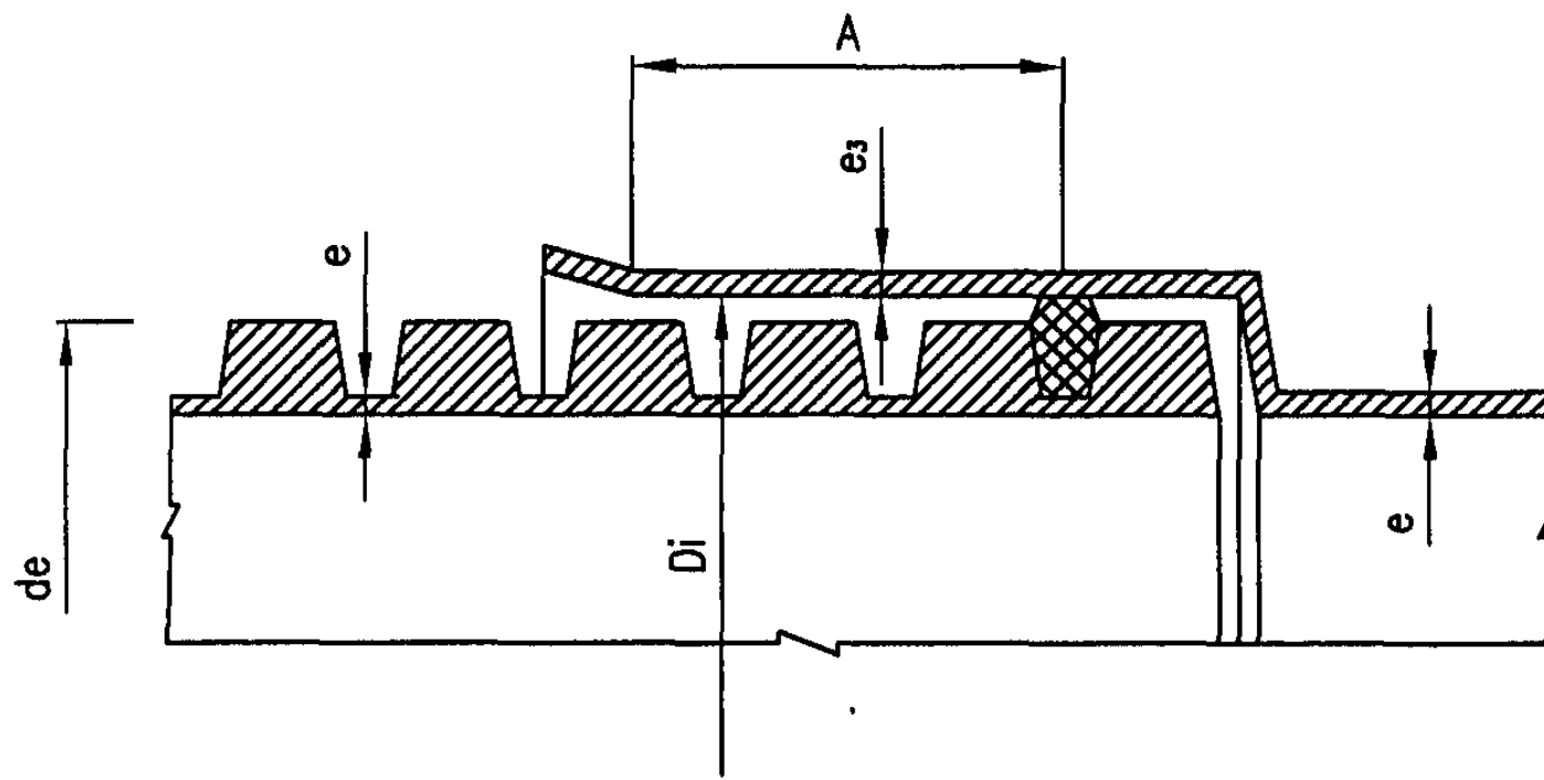
管材承插口
