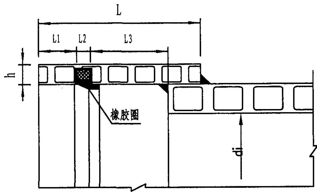
a 雨水管道承口
