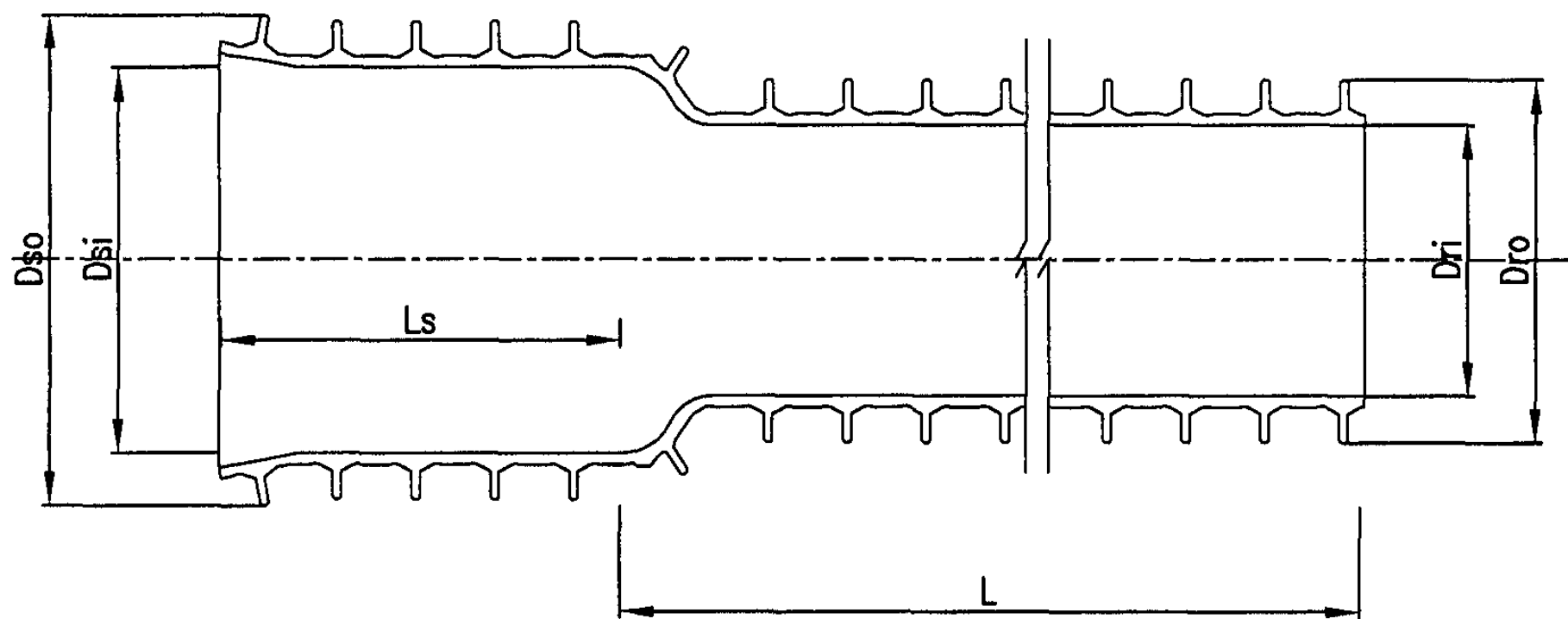
管材规格尺寸
