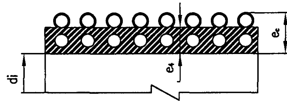
B型结构壁管的典型示例2
