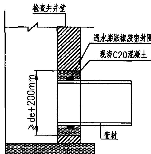
管道与检查井的连接(二)
