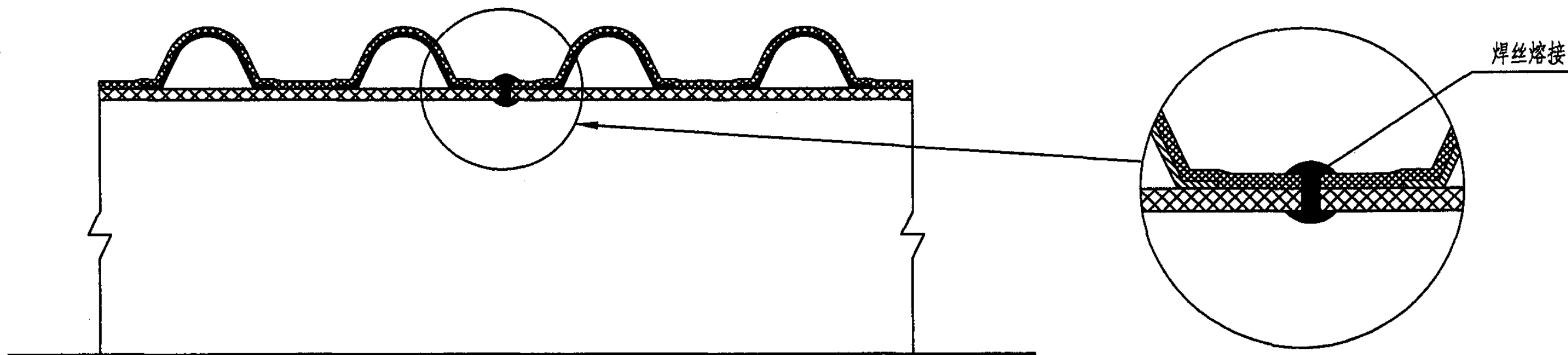
焊接接口示意图
