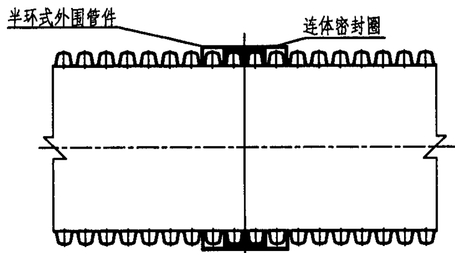
哈夫外固接口
